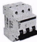
Disjuntor Tripolar 63A Weg Mini DIN MDW C63 5kA Curva C
