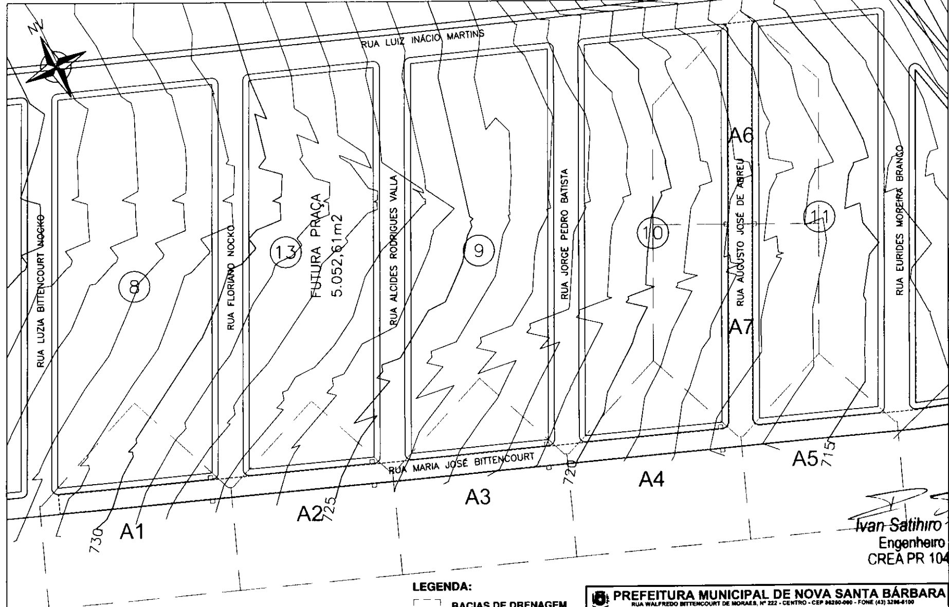
PLANTA BAIXA - BACIAS DE DRENAGEM escala 1:750
