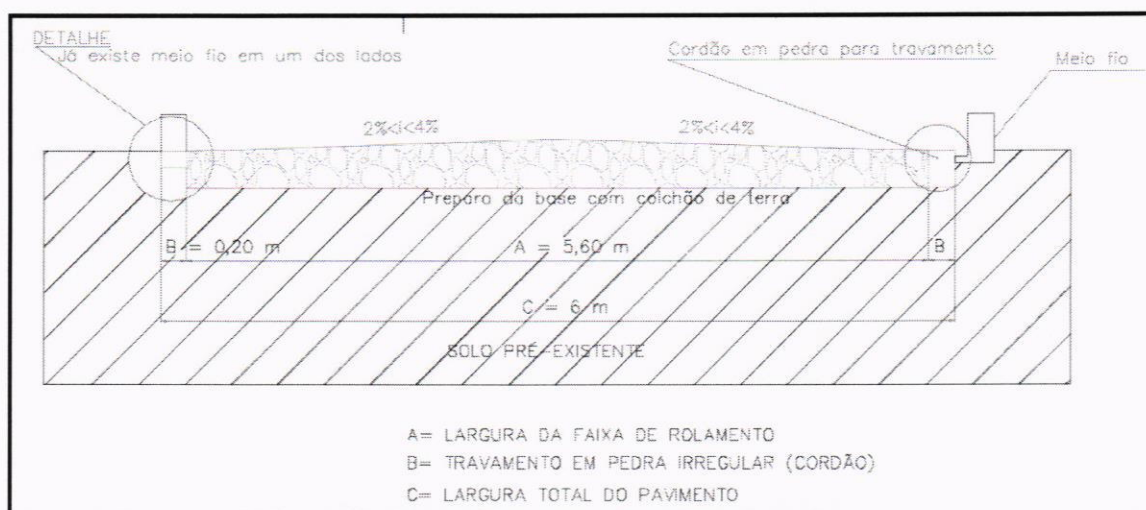
Figura 05: Obra Conjunto América (Projeto inicial) – Corte esquemático
