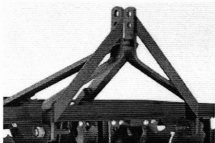
Engate hidráulico categoria I e II. Cat I - II. 3 point hitch. Enganche hidráulico categoría I y II.
